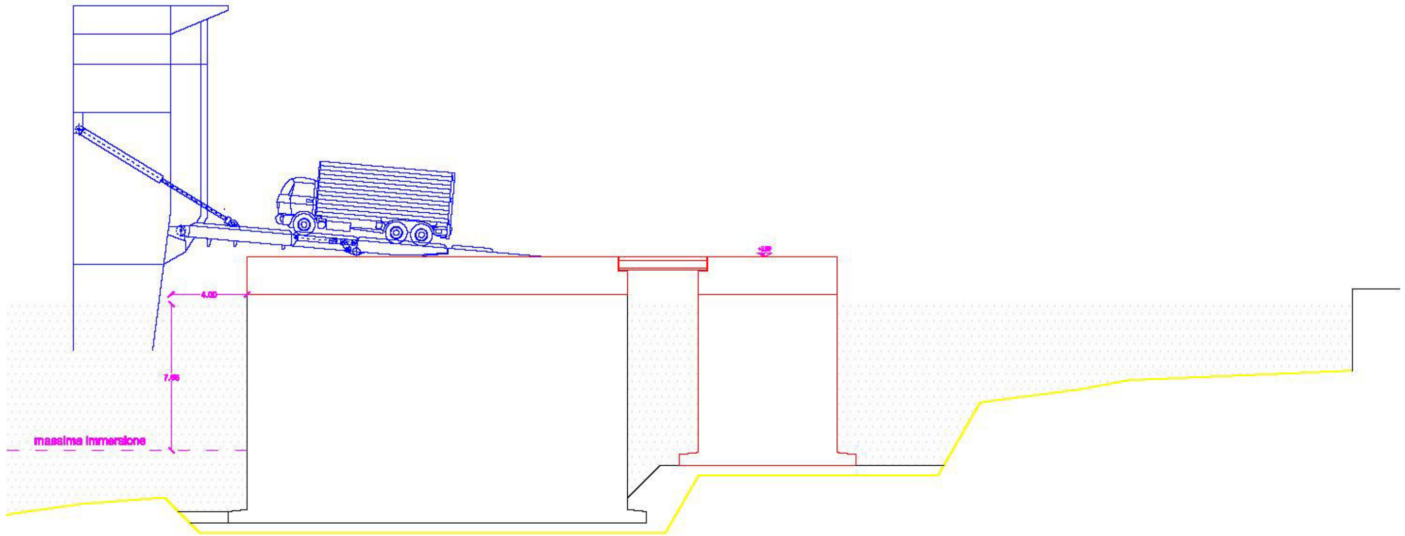
Figura 20 Schema progettuale di carico con mezzo IVECO (non in scala)
