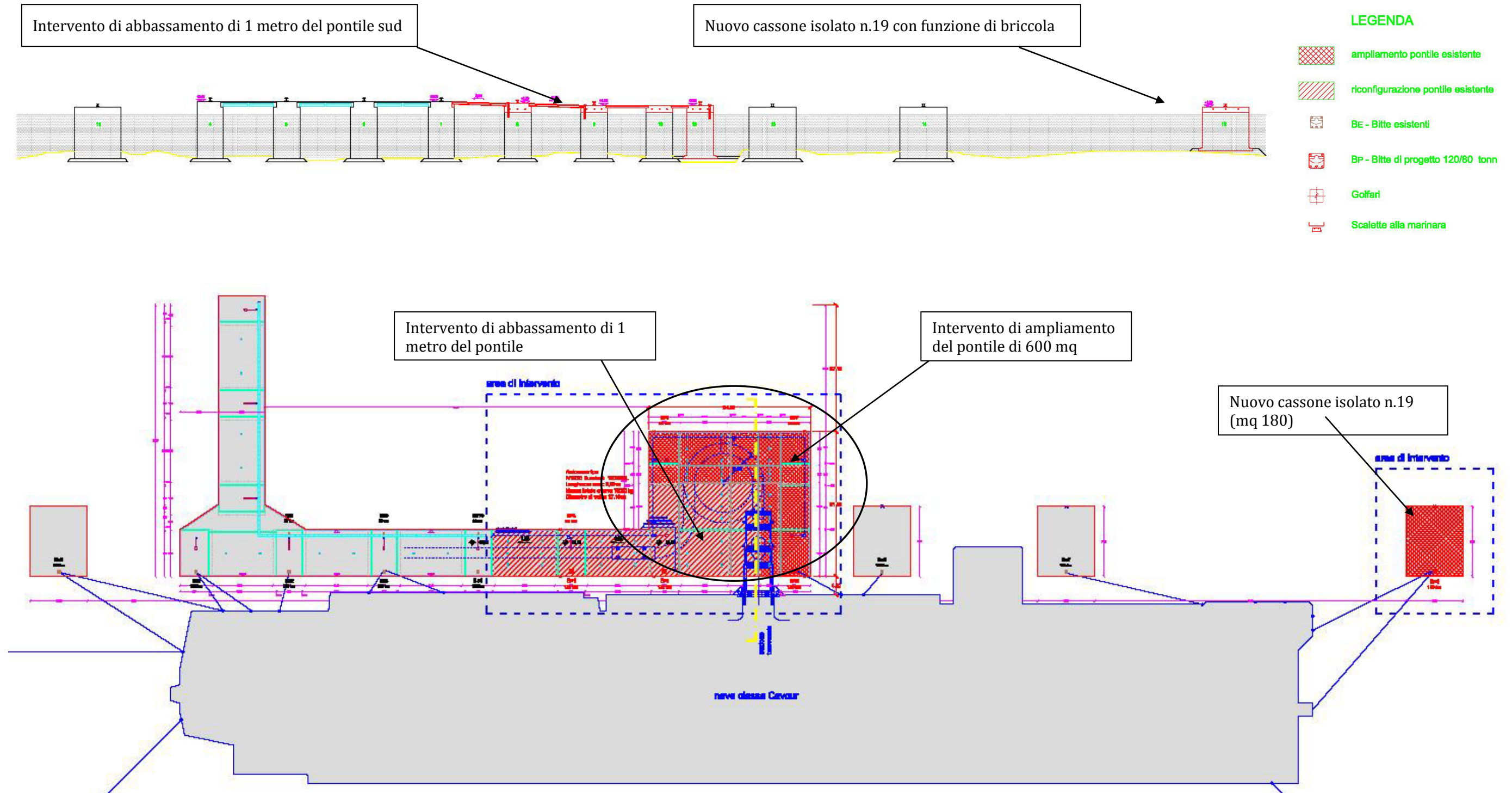
Figura 19 Prospetto e Planimetria intervento di riconfigurazione del pontile sud (non in scala)
